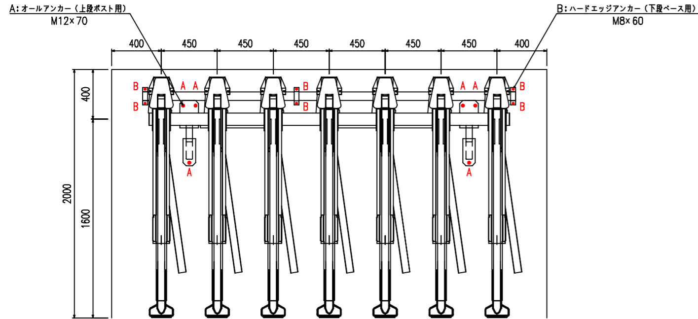
平面図
