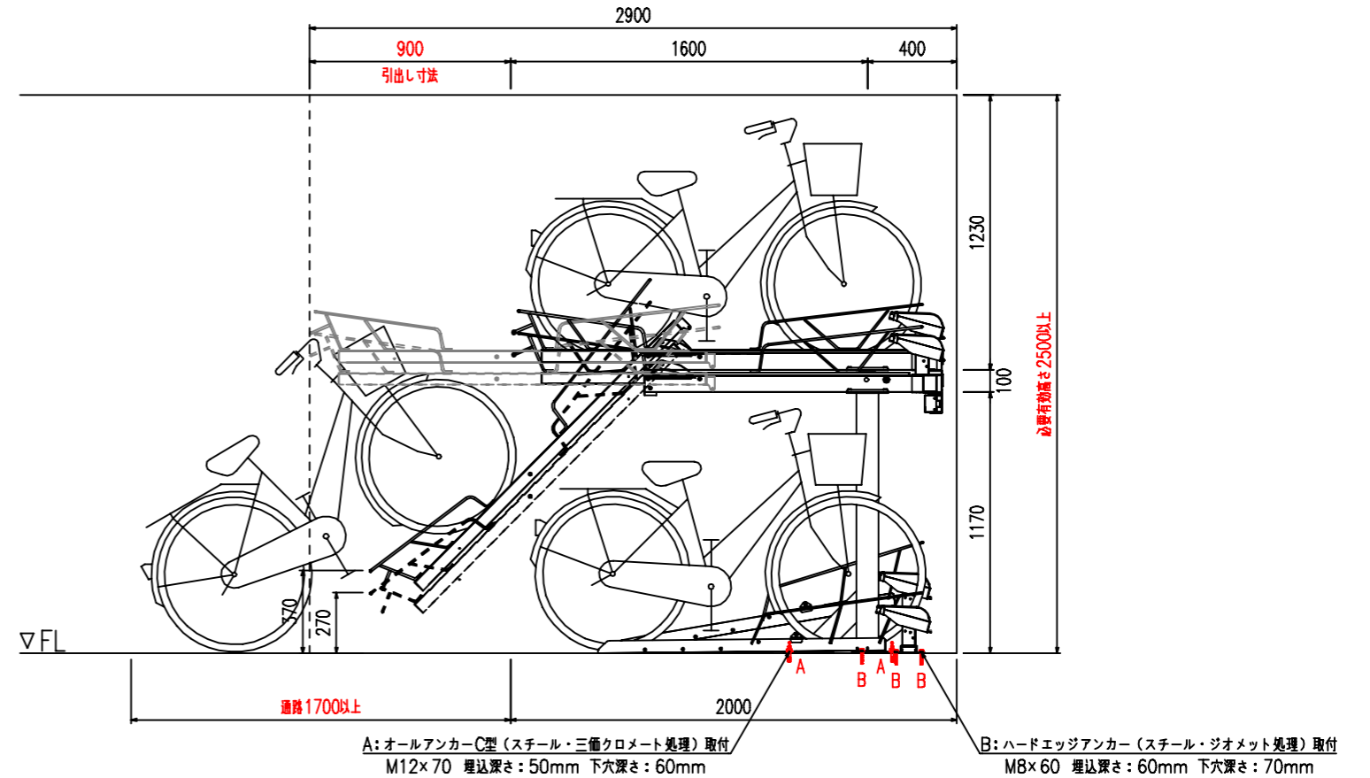
側面図
