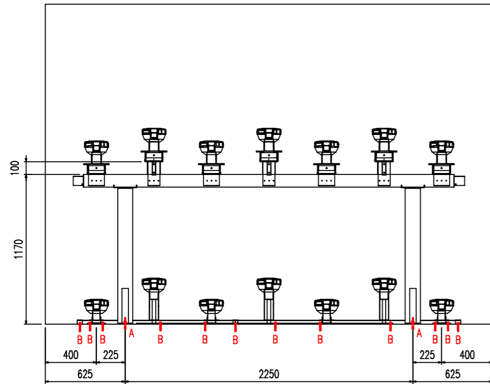
正面図
